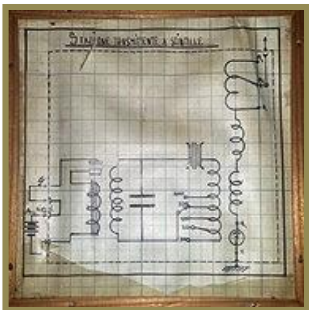
Schema elettrico
