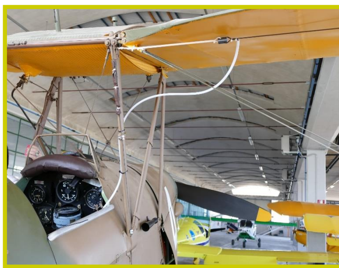
Foto N° 24 tubo di plastica isolante, fascettato sui montanti interalari usato per fare entrare il cavo d'antenna nell'abitacolo
